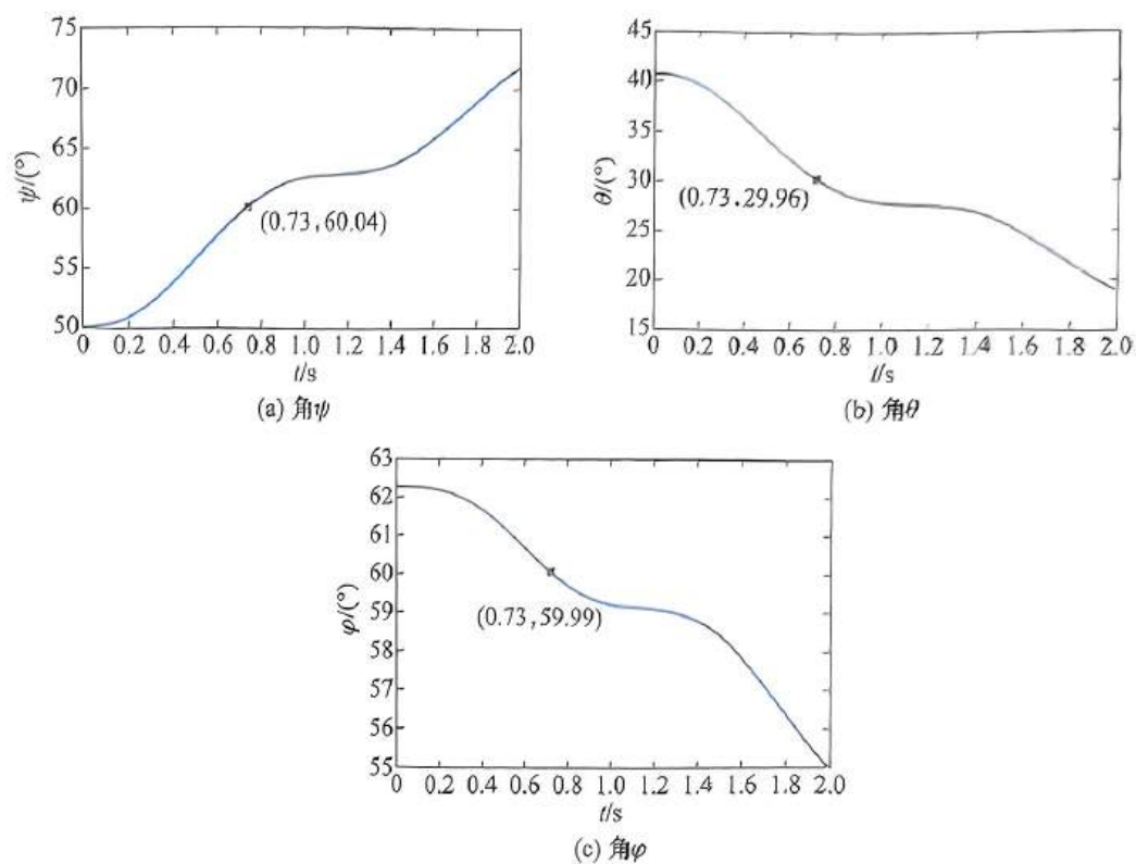
图 1-15 广义坐标随时间变化曲线
