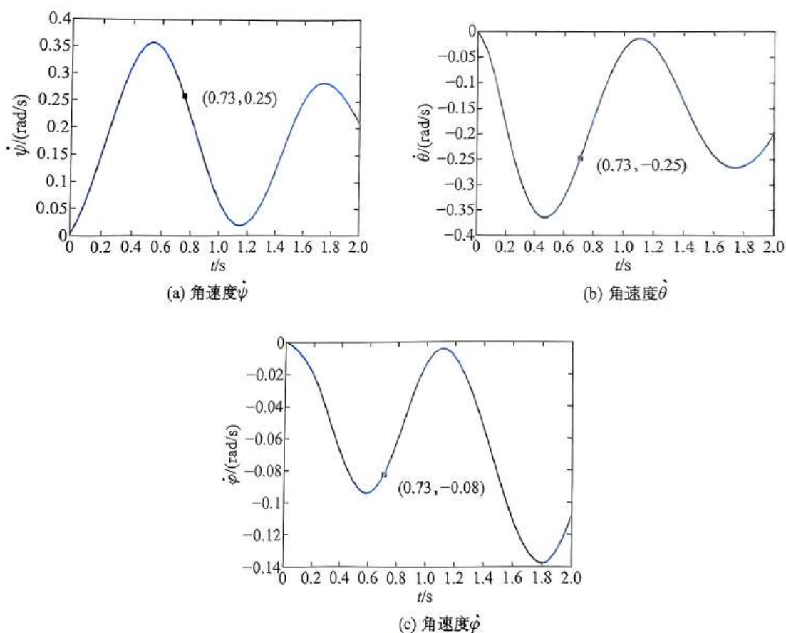
图 1-16 角速度随时间变化曲线
