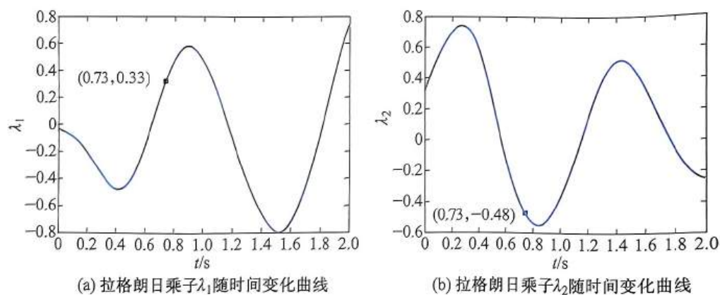
图 1-18 拉格朗日乘子随时间变化曲线
