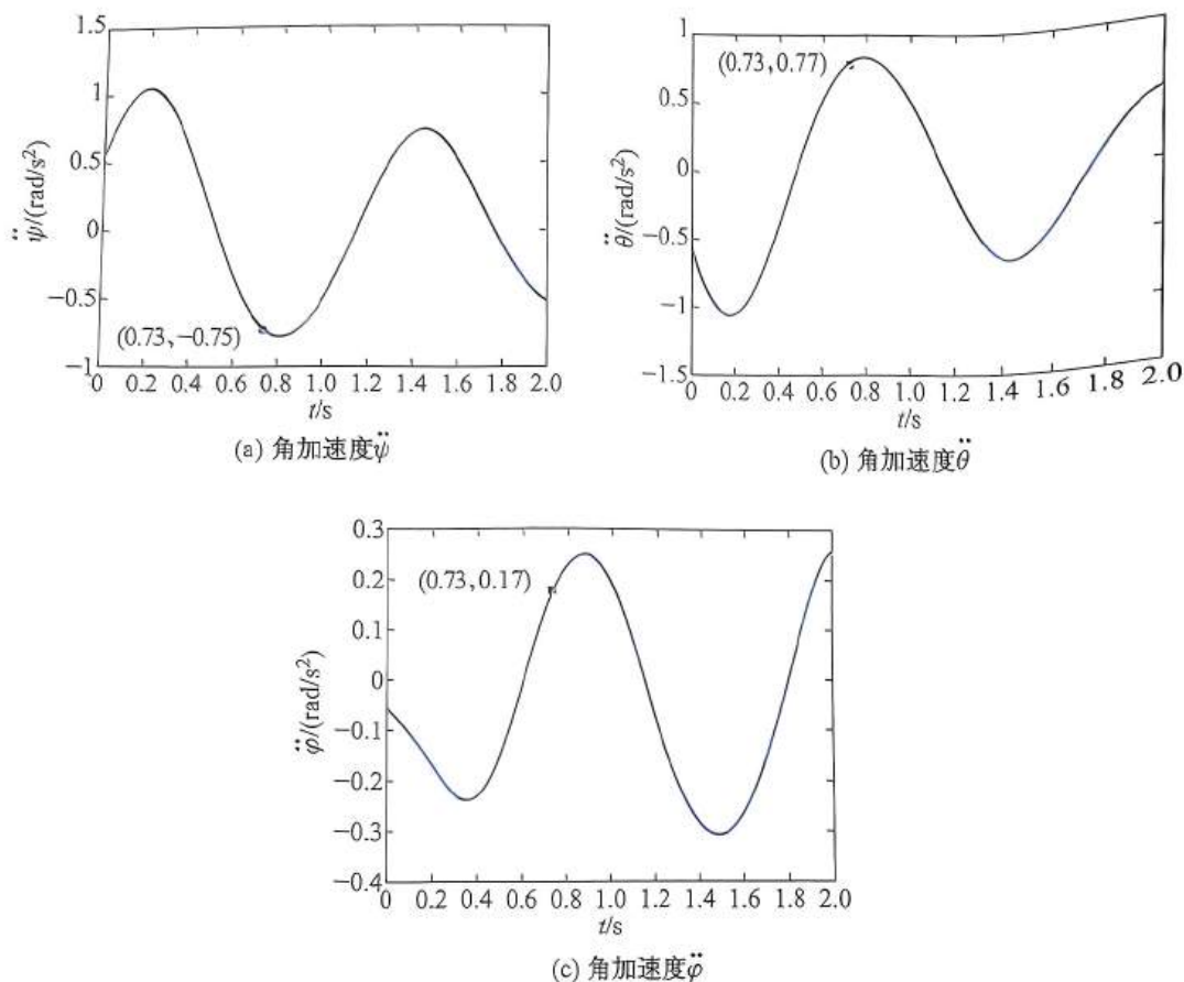
图 1-17 角加速度随时间变化曲线
